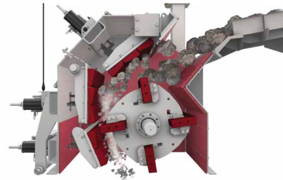
Slika 1: Primarni udarni drobilnik
