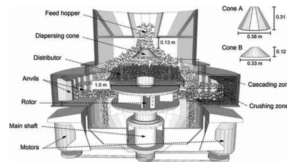
Slika 2: Sekundarni vertikalni udarni drobilnik
