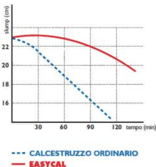
Perdita/mantenimento lavorabilità con temperatura del calcestruzzo di 25 °C
